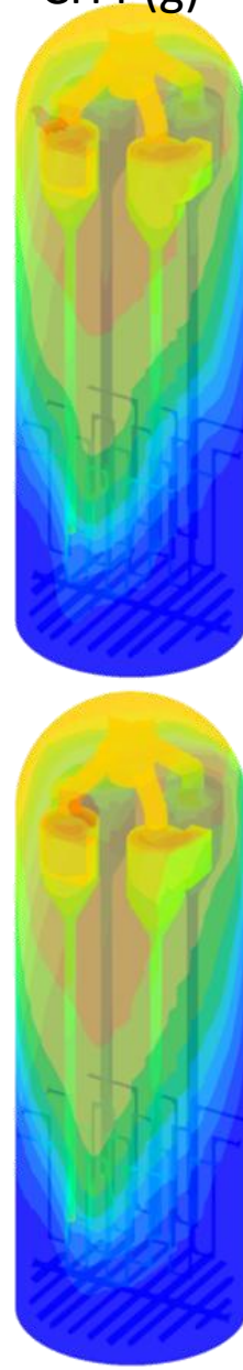
CH 4 (g)
