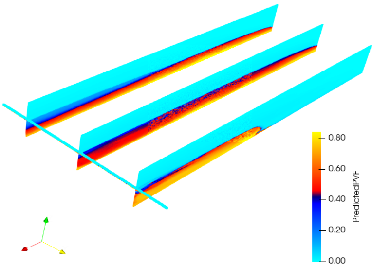
PhysicsNeMo (ROM)
