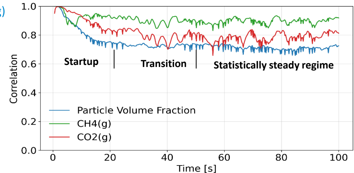
CO2 (g)
