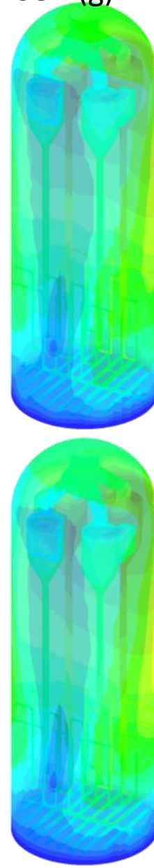
CO 2 (g)
